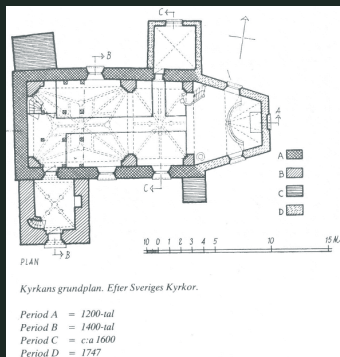
Plan över kyrkan med byggnadsskedena markerade.
